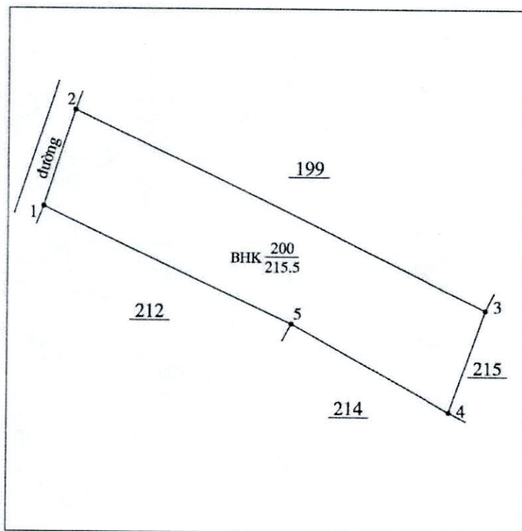
5.1 Sơ đồ thửa đất
